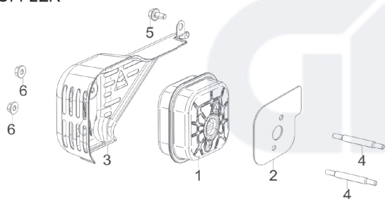
E09 MUFFLER
