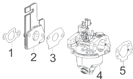
E07 CARBURETOR
